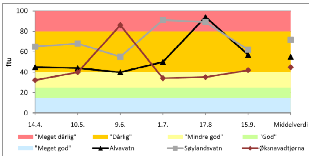
Figur 4.4. Fargetal på dei ulike prøvetakingsstasjonane i 2010, samt aritmetisk middelværdi (snitt). Grenseverdiar for tilstandklassifisering frå SFTs klassifiseringssystem er markert med farga bakgrunn.
