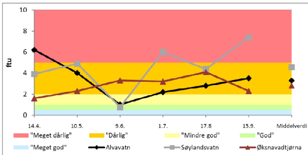
Figur 4.3. Turbiditet på dei ulike prøvetakingsstasjonane i 2010, samt aritmetisk middelværdi (snitt). Grenseverdiar for tilstandklassifisering frå SFTs klassifiseringssystem er markert med farga bakgrunn.
